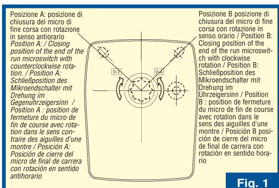
Fig. 1 Vista dalla manopola manuale (vedi fig.2) Rotazione angolare tra adattatore e albero servocomando a gradini di 45° Figure 1. View of the manual knob (see figure 2). Angular rotation between the adapter and a 45-degree step shaft of the servo control. Abb. 1 Ansicht des manuellen Handrads (siehe Abb.2) Eckdrehung zwischen Adapter und Servosystemwelle mit 45°- Stufen Fig. 1 Vue de la manette manuelle (voir fig.2) Rotation angulaire entre adaptateur et arbre servocommande par étape de 45° Fig. 1 Vista del pomo manual (ver fig.2) Rotación angular entre adaptador y árbol de servomando a escalones de 45°
