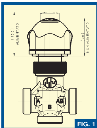
Fig. 1 Applicazione forze serie V3EC Application of forces series V3EC Kraftanwendung Baureihe V3EC Application des forces série V3EC Aplicación fuerzas serie V3EC
