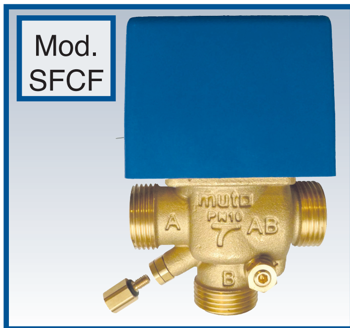
Die Ventile sind mit einem externen Hebel für die manuelle Positionierung des Verschlusses in die zentrale Position (Abb. 3) versehen. Außerdem verfügt die Version PLUS über einen regulierbaren Bypass und über einen manometrischen Druckstecker, um den Hydraulikkreis bei geschlossenem Ventil auszugleichen.
